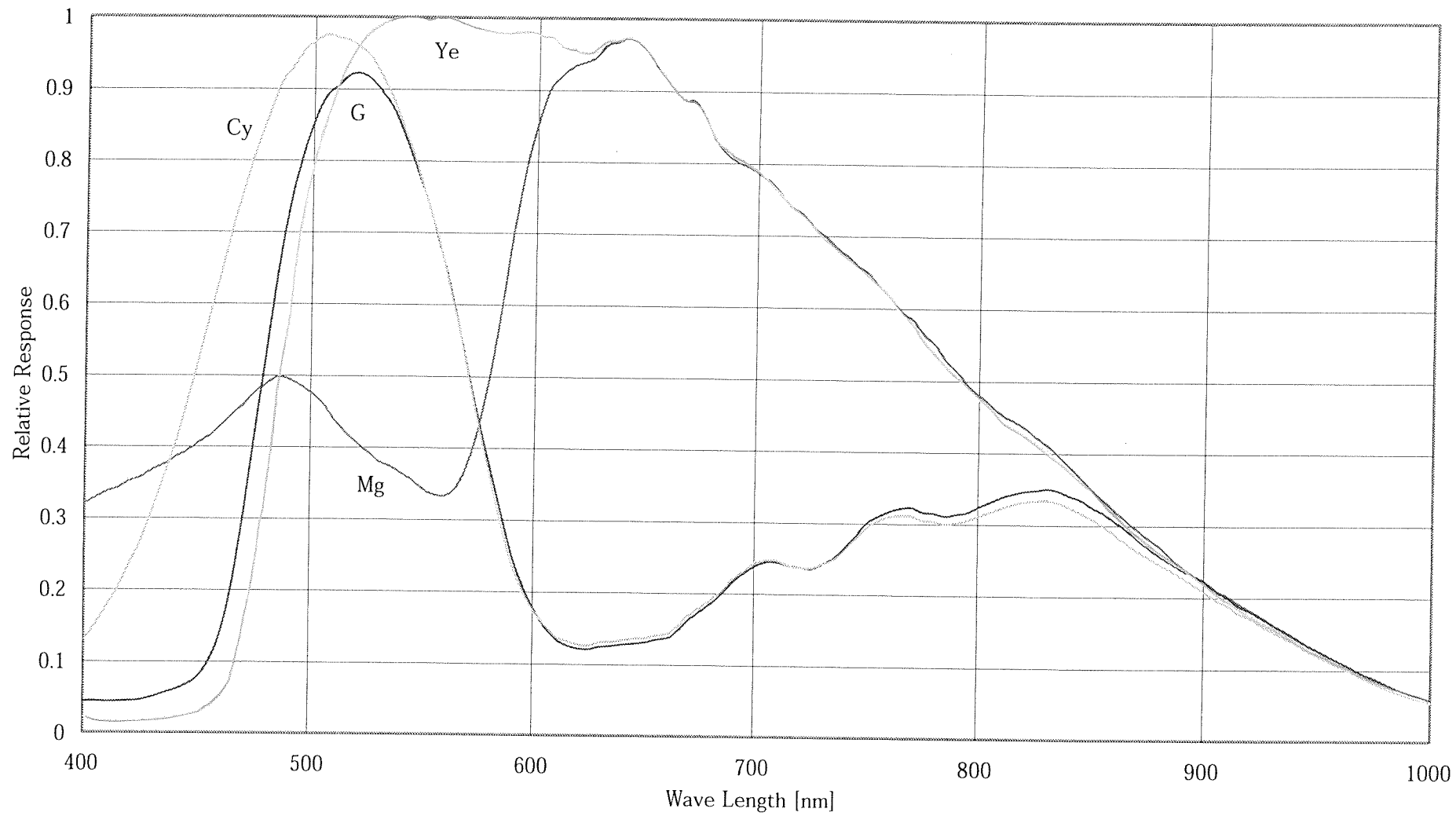
ICX278AK 分光感度特性例
