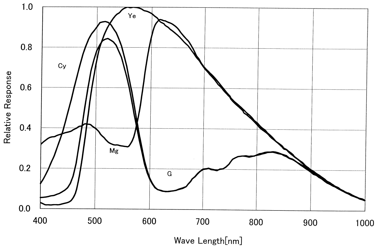
ICX279AK 分光感度特性例 (ただし, レンズ特性および光学特性を除く)
